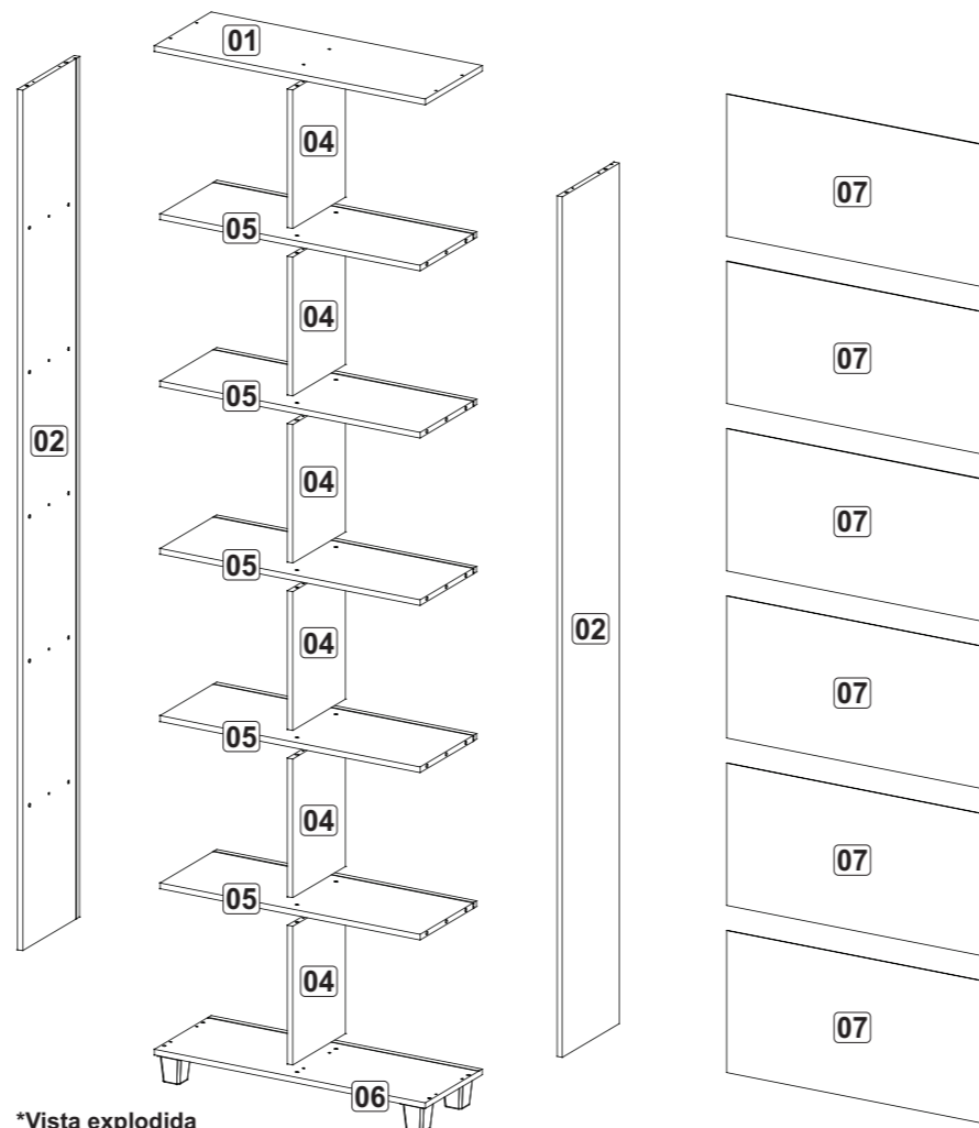
*Vista explodida
