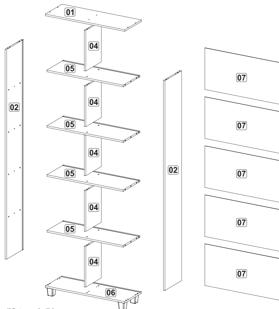
*Vista explodida
